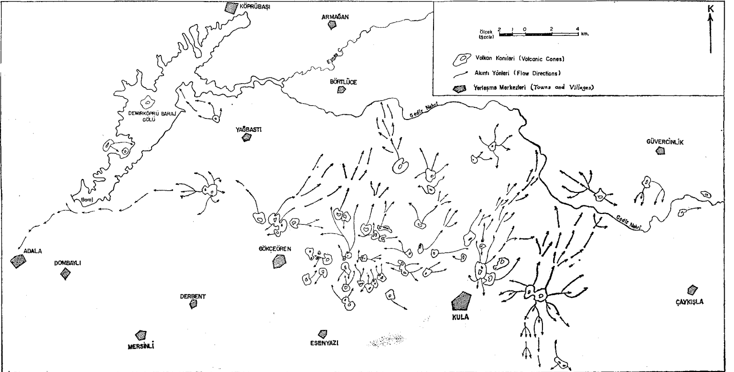
Şekil 2 : Kula lavlarının akıntı yönleri. Figure 2 : Flow directions of Kula lavas.
