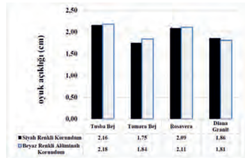
Şekil 9. İki farklı aşındırıcı toz ile yapılan GDA deneyi sonuçları (14 kg'lık sıkıştırma yükünde).
