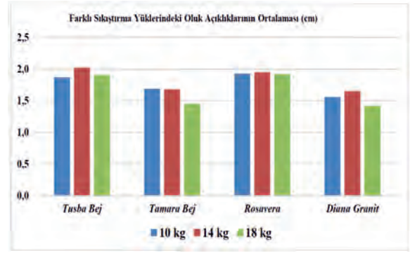
Şekil 7. Farklı sıkıştırma yüklerinde oluşan düzeltilmiş oluk açıklıklarına (DOA) ait ortalama değerleri gösteren bar diyagramı.
