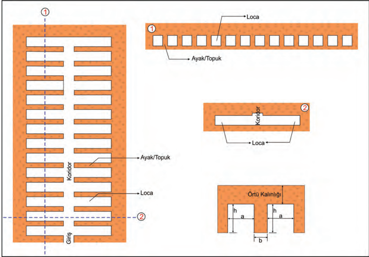
Şekil 3. Tipik bir kaya oyma deponun plan ve kesit görünüşleri.
