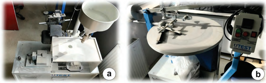
Şekil 3. Geniş Diskli Aşındırma (a) ve Böhme Aşındırma (b) cihazlarına ait bir görüntü.
