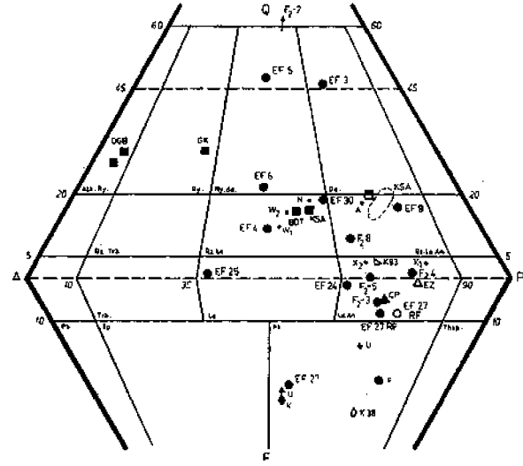
Şekil 2: Foça, Menemen ve öteki bazı Batı Anadolu volkanitlerinden örnek kayaların, çeşitli normlara göre Streckeisen üçgenindeki yerleşimi. Figure 2: The representative specimens «rom Foça, Menemen and other localities of W-"Anatolia, calculated to different norms plotted in Streckeisen's doubletriangle.
