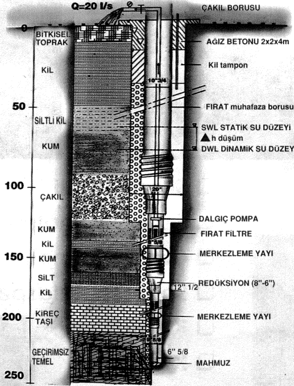
DERİN KUYU ÖN PROJESİ
