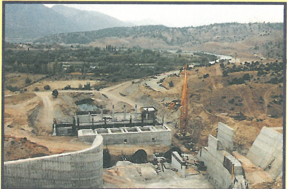
Beyköy HES Santral Binası ve İsale Kanalı İnşaatı
