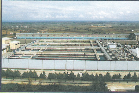
Samsun İçmesuyu Arıtma Tesisi Q=200.000 \text{ m}^3/\text{gün}
