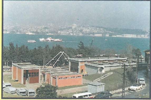
Üsküdar Atıksu Ön Arıtma Tesisi Q=179.000 \text{ m}^3/\text{gün}
