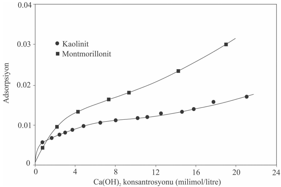
Şekil 4. 25 °C sıcaklıkta montmorillonit ve kaolinit killlerinde gözlenen \text{Ca(OH)}_2 adsorpsiyon eğrileri (Diamond ve Kinter 1966' den değiştirilmiş).
