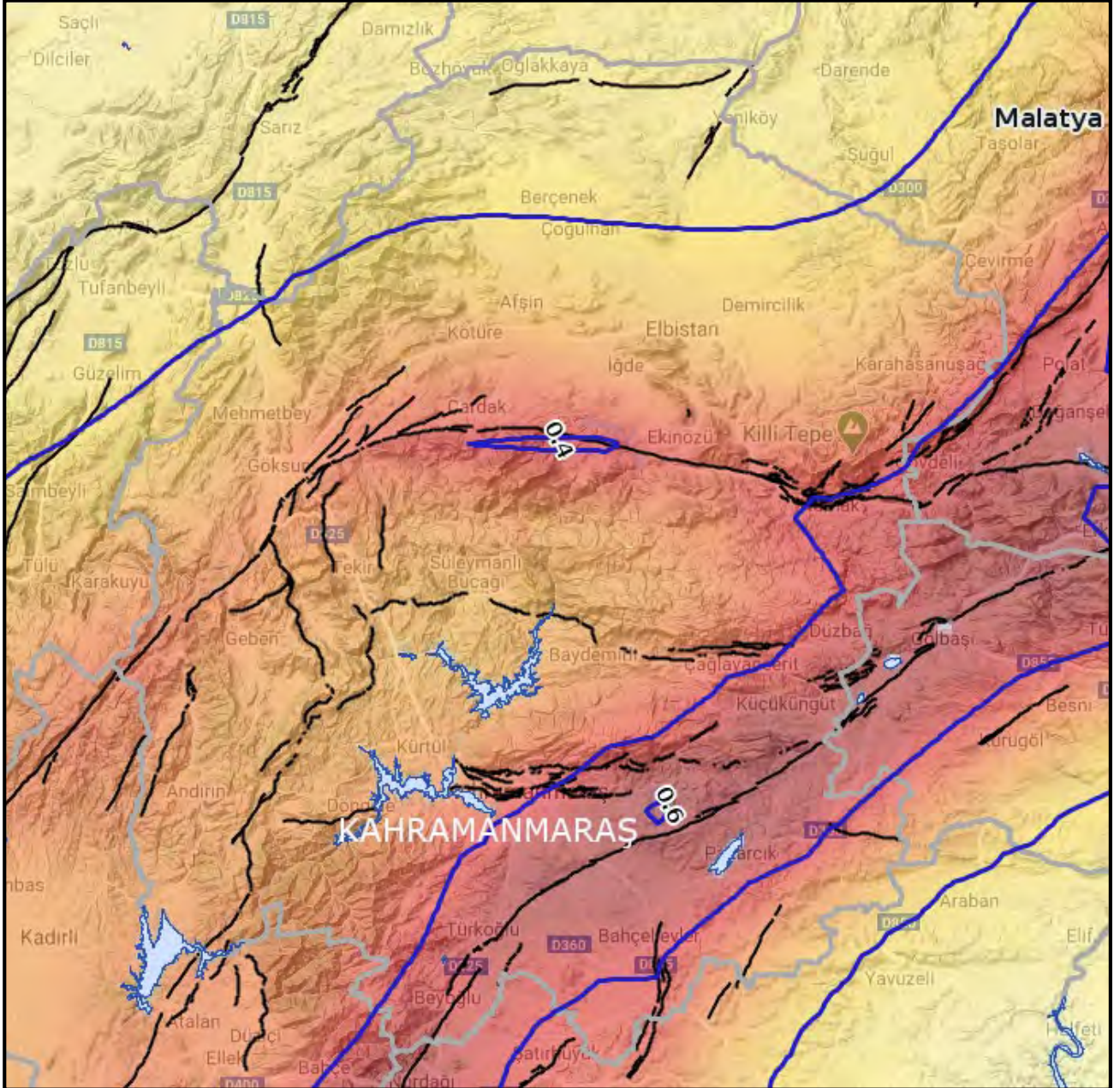
Şekil 1- Kahramanmaraş Deprem Tehlike Haritası ( https://tdth.afad.gov.tr/TDTH/main.xhtml )
