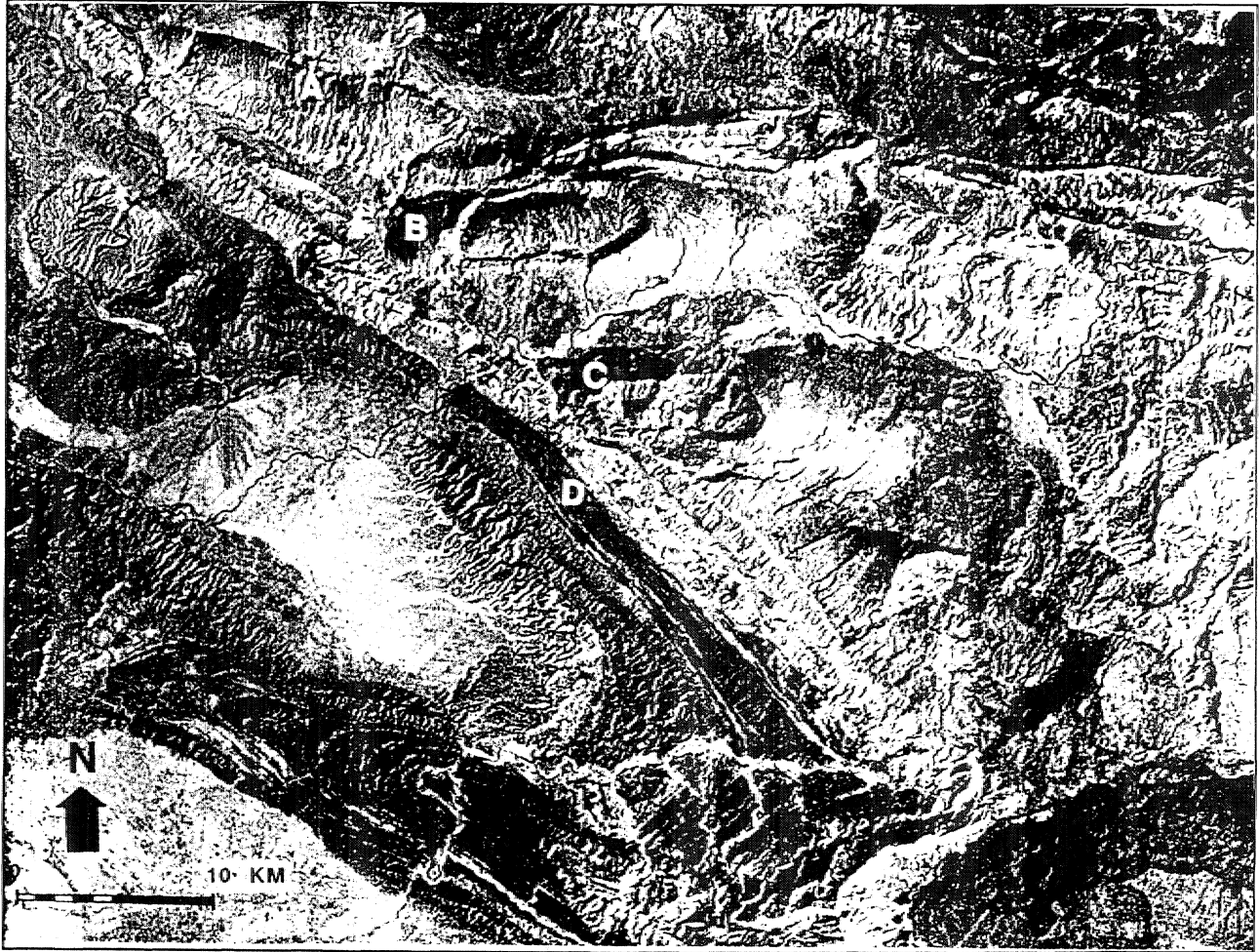
Şekil 9: Süleyman Sıradağları güney kesiminin bu Landsat görünümü, yığınlanma^ antiklinallerde yüzlek veren kesit tekrarını göstermektedir (A,B,C), bir yırtmaç fayı/monoklinal eğilti (D) ve bindirmeye doğru kavis yapan bir yırtmaç fayı (E). (SPOT Image Corp. 1990).
