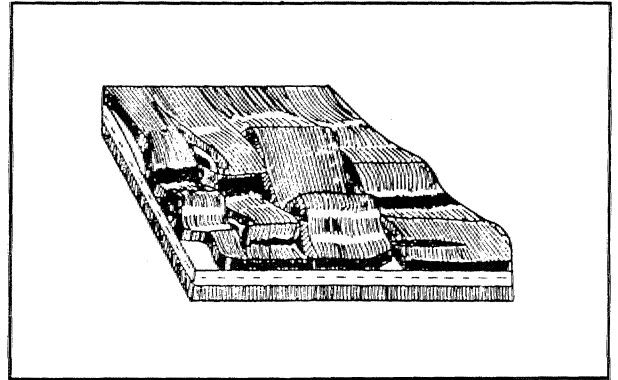
Şekil 6: Bindirme/kıvrım alanlarında, yırmaç fayları şekilde görüldüğü gibi ön bindirmenin içine kavislenebilirler. Kıvrımlar, yırmaç fayının herhangi, bir kenarı üzerinde zıt yönlü olabilirler.. Hareket eğim-aüm ya da doğrultu-atımlı görün ebilir. Bindirme fayları, doğrultuları boyunca hareketlerini kıvrımlanmaya transfer ederler.
