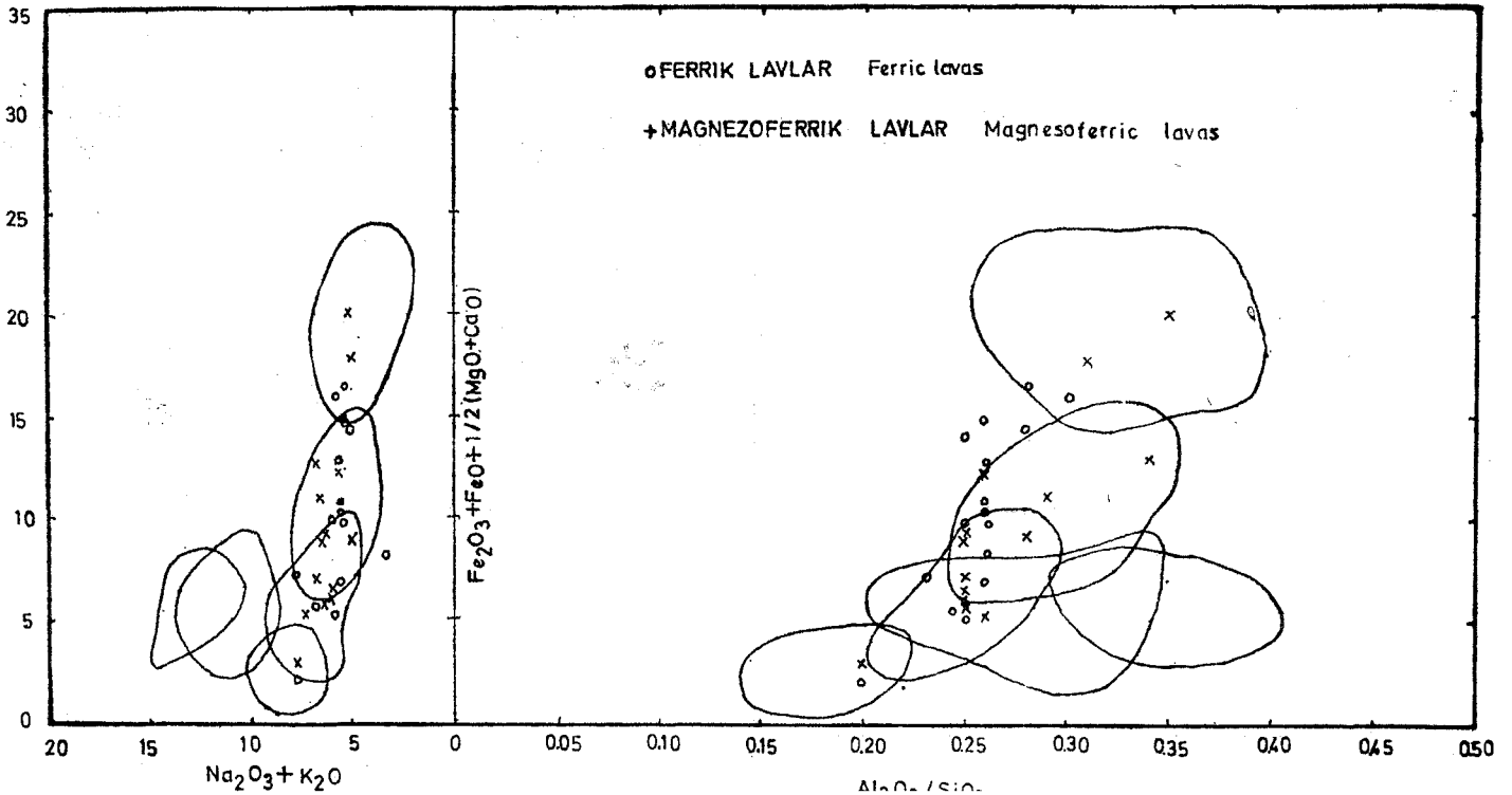
Şekil 4: Kızılcahamam güneybatısındaki lavların niceliksel sınıfla
