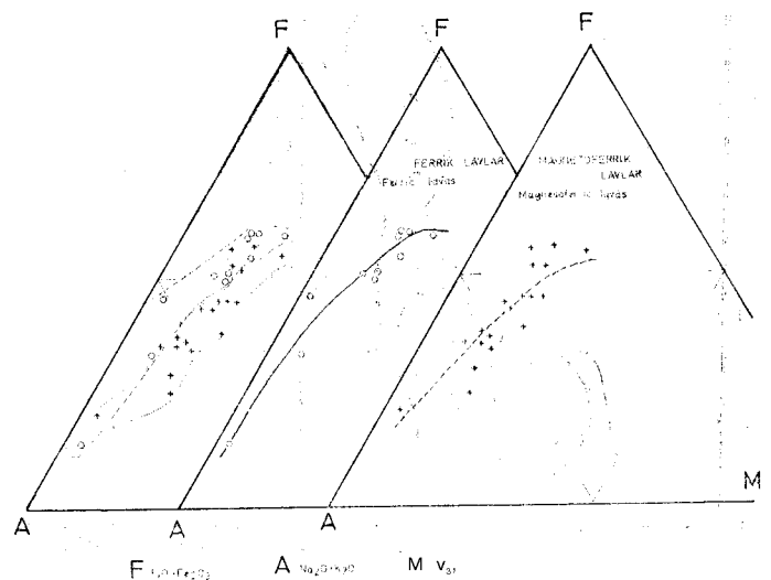
Şekil 7: Kızılcahamam güneybatısındaki lavaların FAM eğrisi.
