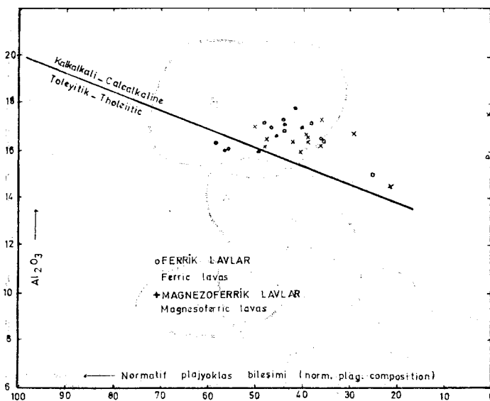
Şekil 6: Kızılcahamam güneybatısındaki lavaların Al_2O_3 /normatif plajyoklas eğrisi.
