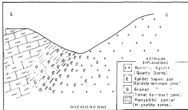
Şekil 4 Skarlarda zonlanma (ölçeksiz). Figure 4 Zonation of skams (no scale).
