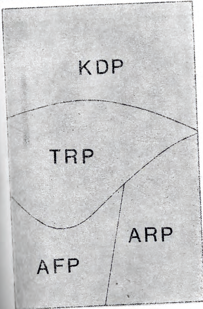
Şekil 4: KAF'a komşu plakaların analitik modeli: a) plaka sınırları, b) modelin sonlu elemanlara bölünümü. Figure 4: The analytical model of the plates adjacent to the NAF: a) plate boundaries, b) finite element idealization of the model. KDP : Karadeniz plakası — Black Sea Plate TRP : Türkiye Plakası — Turkish Plate AFP : Afrika Plakası — African Plate ARP : Arap Plakası — Arabian Plate
