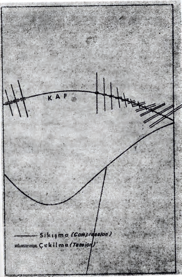
Şekil 6: KAF boyunca belirli bazı noktadaki en büyük ve en küçük asal gerilimler.
