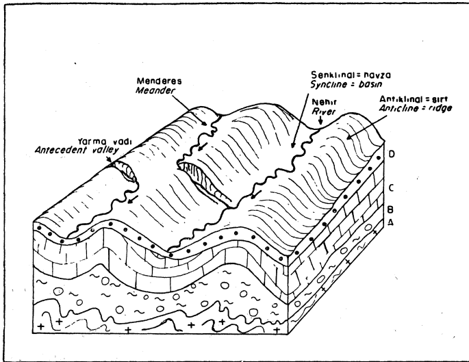
Şekil 2 : Doğu Anadolu'nun neotektonik dönemdeki yapı - morfolojisi ilişkilerini gösteren blok diyagramı.
