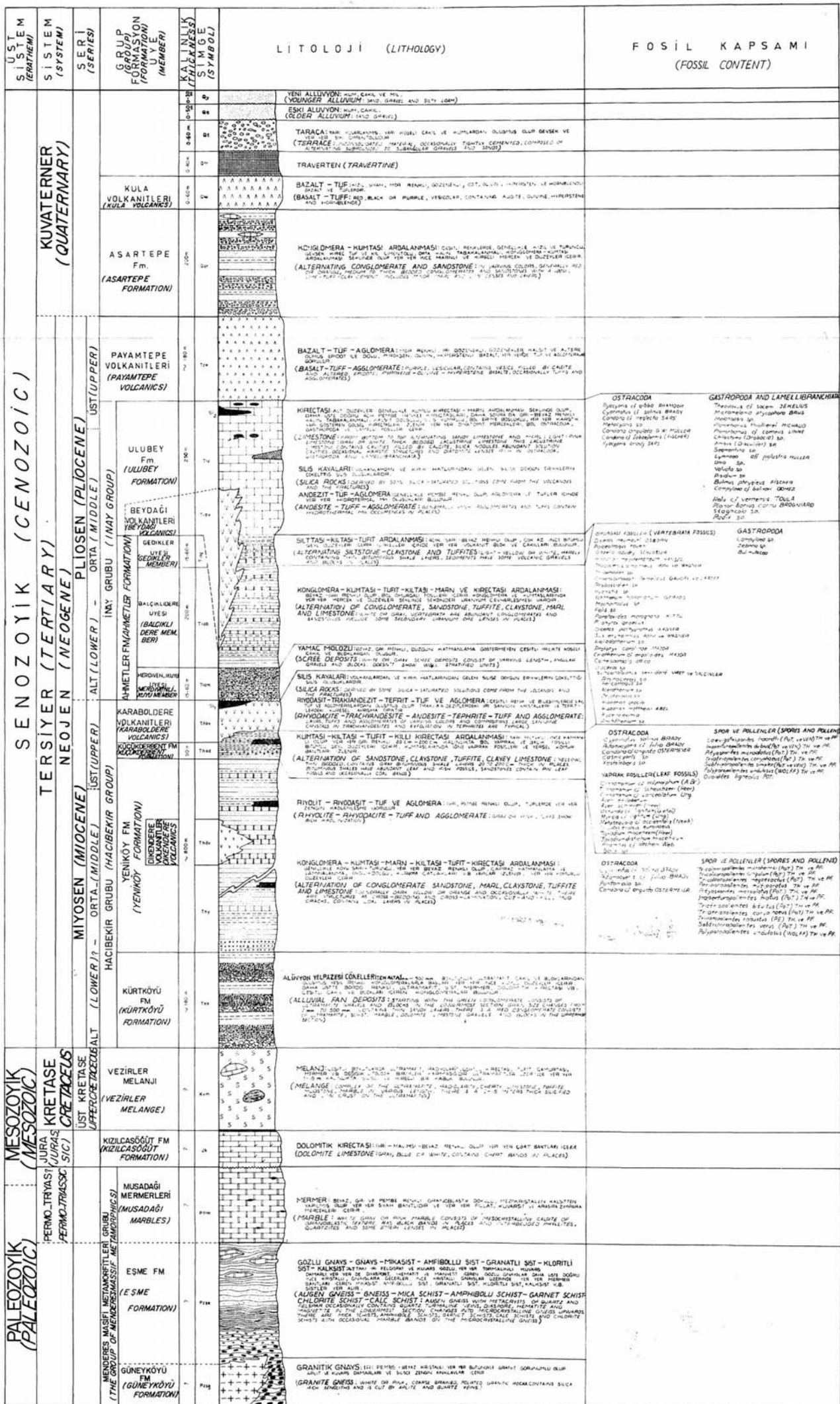
Sekil 2: İncelenen alanın genelleştirilmiş dilme kesiti. Figure 2: Generalized columnar section of the investigated area.
