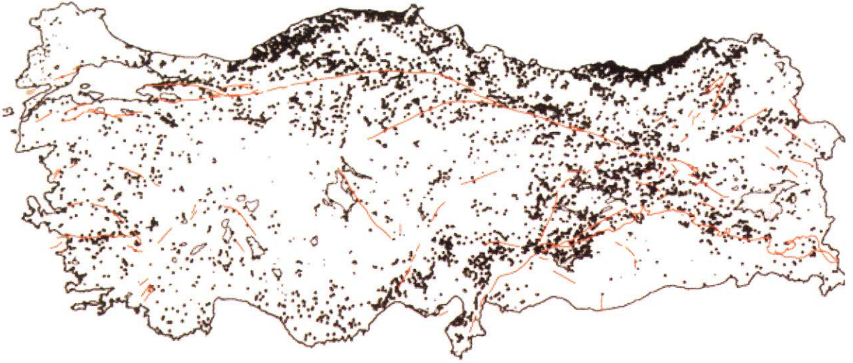
Şekil 2-Türkiye’de heyelanlı yerleşim birimlerinin yersel dağılımının aktif faylarla ilişkisi (1).
